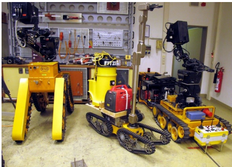
Verschiedene Manipulatoren der KHG
